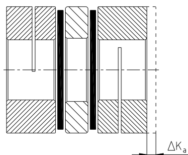
odchyłka osiowa
