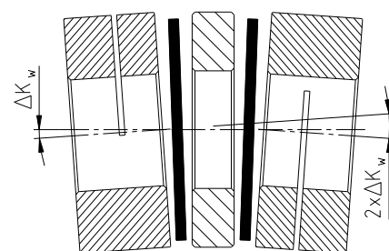
odchyłka kątowa
