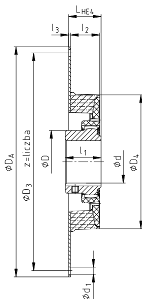
rysunek 4: BoWex-ELASTIC® typ HE4
