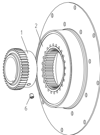
rysunek 9: BoWex-ELASTIC® typ HE4
