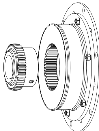
wykonanie HE2
