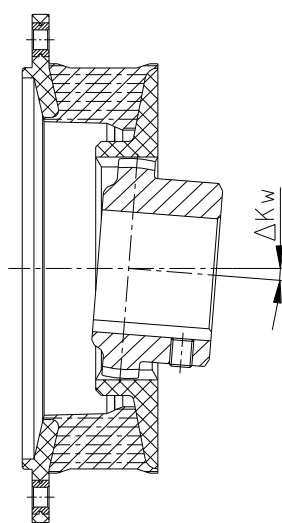
odchyłka kątowa
