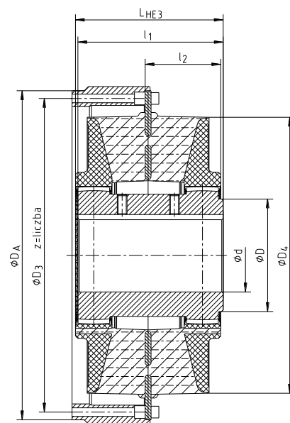
rysunek 5: BoWex-ELASTIC® typ HE-D
