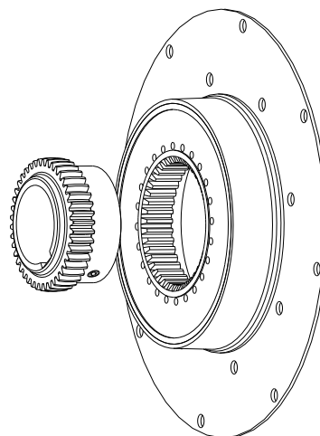
wykonanie HE4
