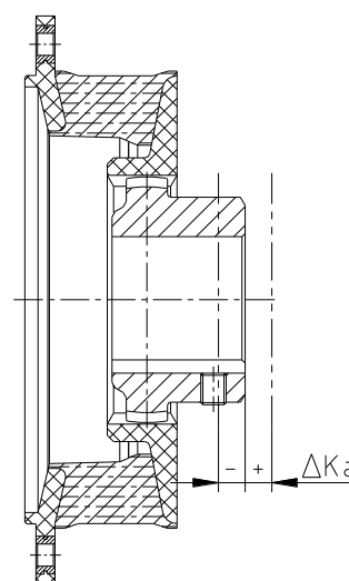
odchyłka osiowa
