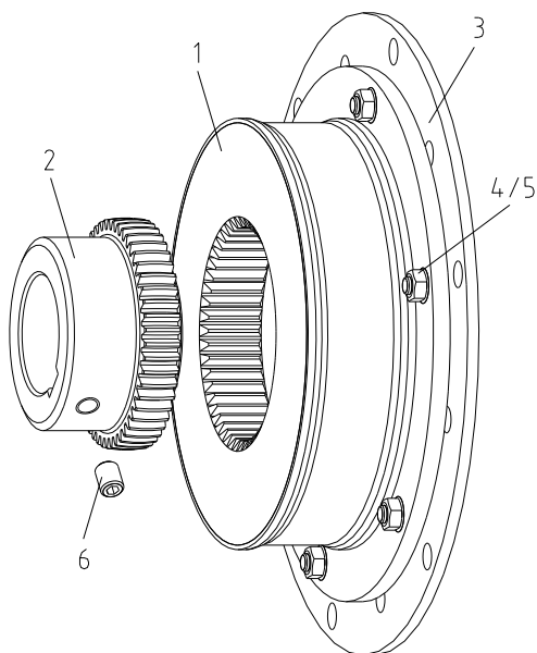
rysunek 6: BoWex-ELASTIC® typ HE1
