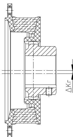
odchyłka promieniowa
