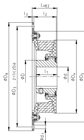
rysunek 2: BoWex-ELASTIC® typ HE2
