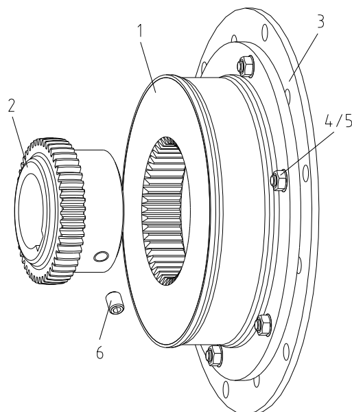
rysunek 7: BoWex-ELASTIC® typ HE2
